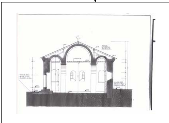
попечни пресек
