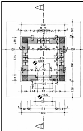
основа звоника
